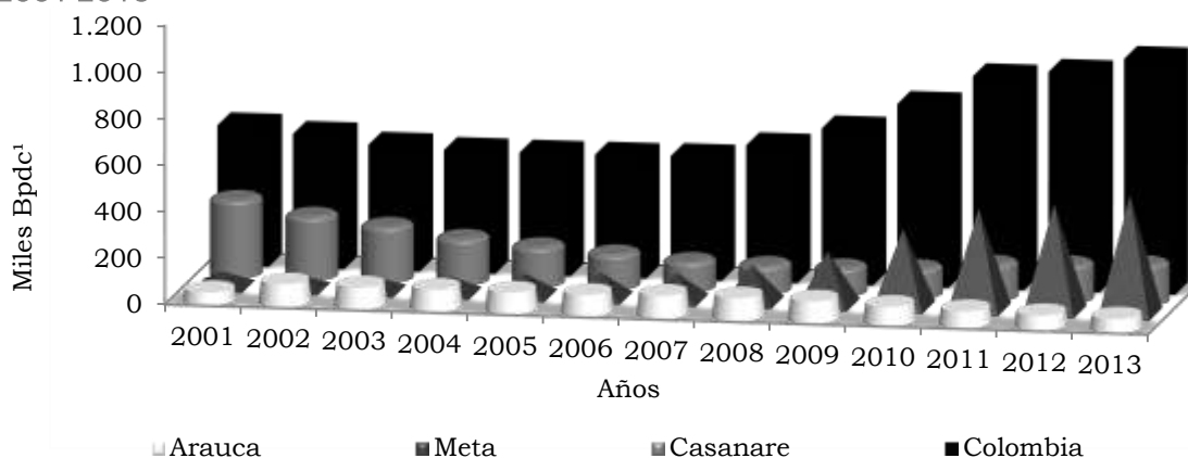
Gráfico 3.4.3.1. Colombia-Arauca-Meta-Casanare. Evolución promedio de la producción petrolera 2001-2013
