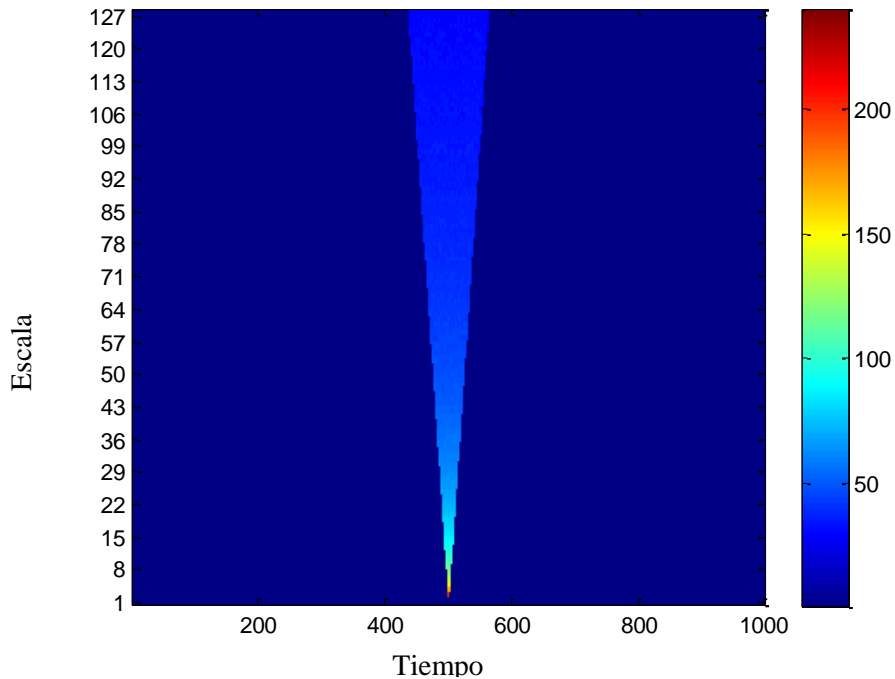
Gráfico 3. Valor absoluto de los coeficientes wavelet
