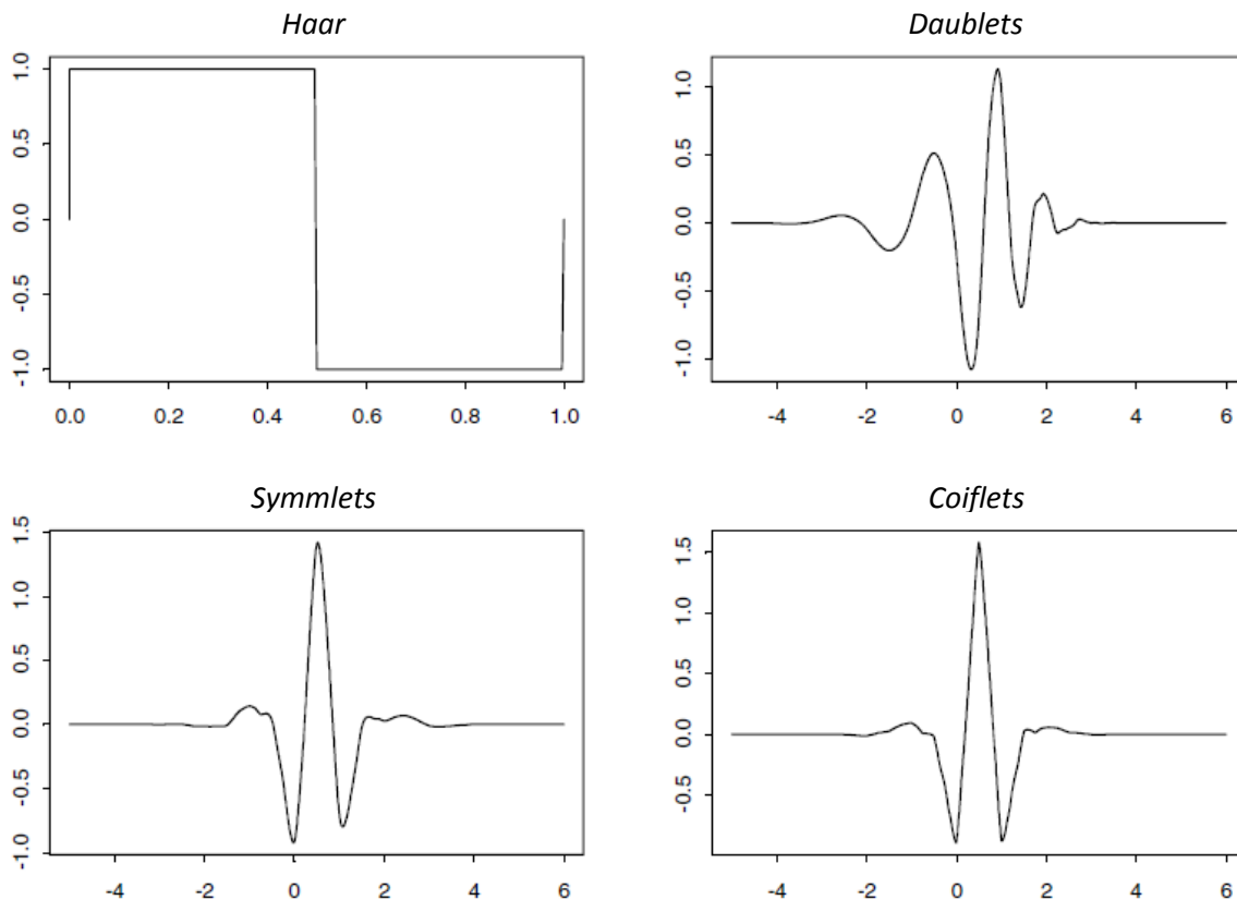
Gráfico 1. Ejemplos de funciones wavelet
