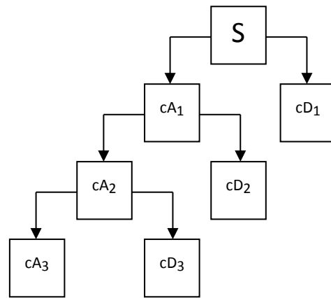
Gráfico 5. Análisis Multi-resolución 19
