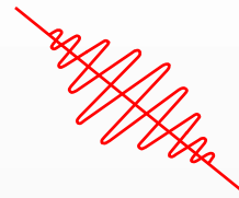
Firewall SEBRA
