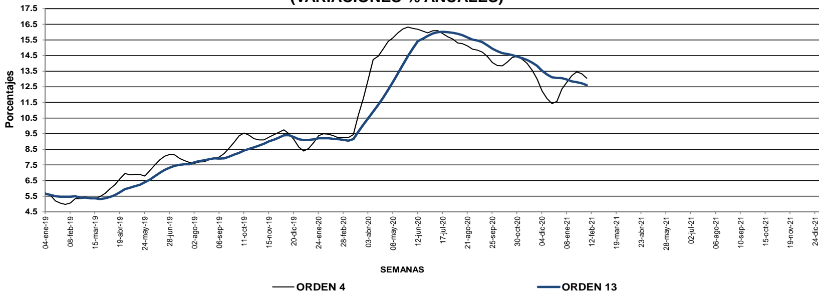
GRAFICO 8 M3* PROMEDIOS MOVILES DE ORDEN 4 Y ORDEN 13 (VARIACIONES % ANUALES)
