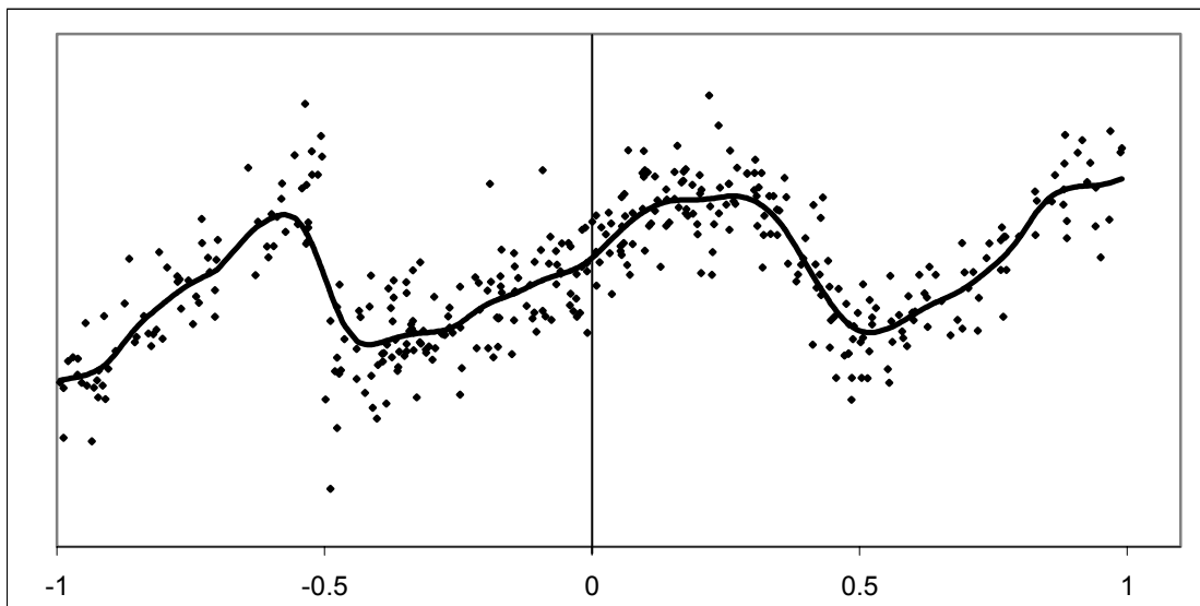
Gráfico 4. Estimación kernel, con h optimo, h=0.1527.
